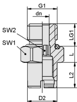
Datos de diseño SC-A 045 G3/8-AG L
