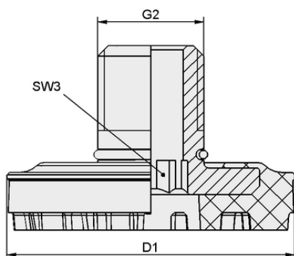
Конструктивные данные SC-S 055 FDC-L
