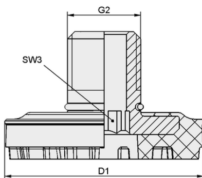
Données de construction SC-S 055 FDC-L
