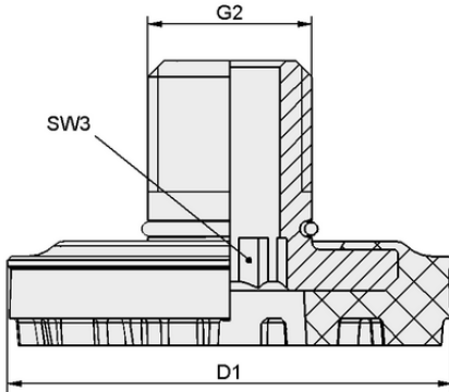
Tasarım verileri SC-S 045 FDC-L
