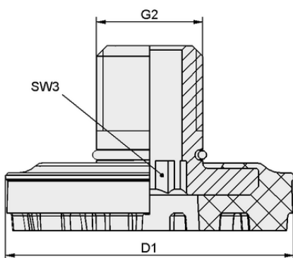
Datos de diseño SC-S 045 FDC-L
