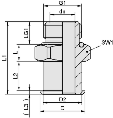
Tasarım verileri SC 090 G1/4-AG
