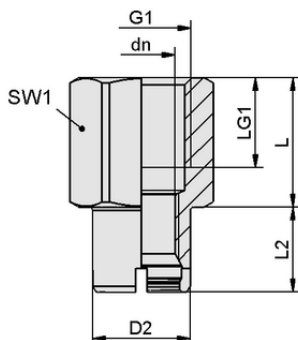
Datos de diseño SC-A 065 G1/4-IG L
