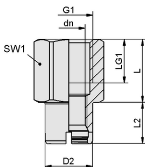
Конструктивные данные SC-A 065 G1/4-IG L
