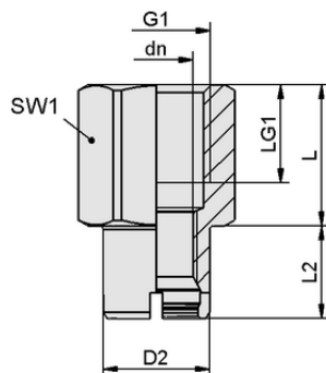
Datos de diseño SC-A 055 G3/8-IG L
