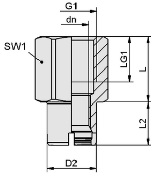
Tasarım verileri SC-A 055 G1/4-IG L
