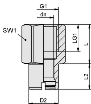
Конструктивные данные SC-A 045 G3/8-IG L
