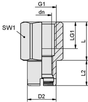
Tasarım verileri SC-A 045 G1/4-IG L
