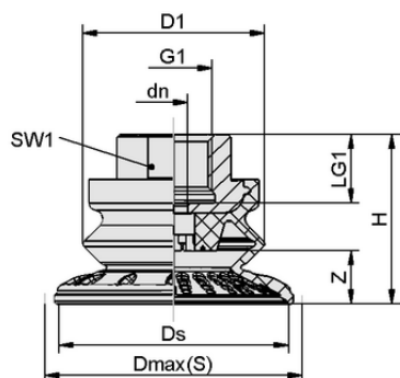
デザインデータ SAB 125 HT1-60 G3/8-IG
