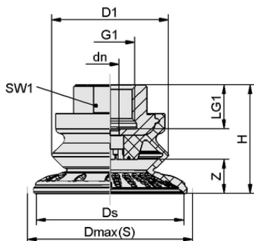
Données de construction SAB 30 HT1-60 G1/4-IG
