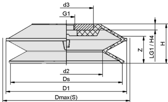
Datos de diseño FSGPL 150 NBR-55 G1/2-IG C
