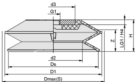
Dati di costruzione FSGPL 150 NBR-55 G1/2-IG C
