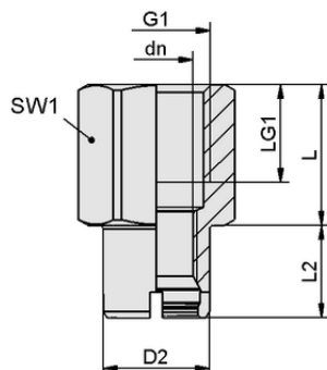
Конструктивные данные SC-A 065 G3/8-IG L
