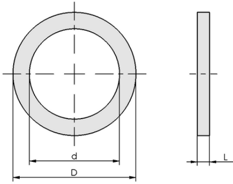
Tasarım verileri DR 78/54x5 MOS SI-15
