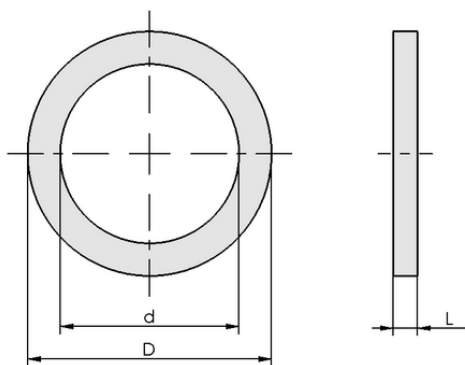
Dati di costruzione DR 42/20x5 MOS SI-15
