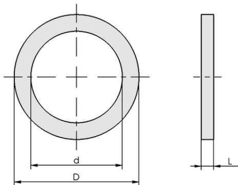
デザインデータ DR 22.5/13x2 MOS SI-15
