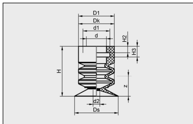
Datos de diseño FG 19 NK-45 N047
