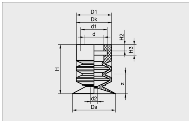
Dati di costruzione FG 19 NK-45 N047
