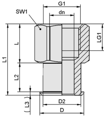
Tasarım verileri SC 080 G3/8-IG
