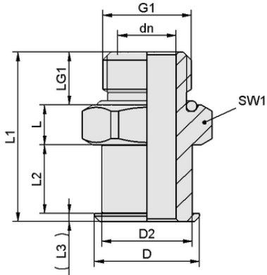
Tasarım verileri SC 080 G3/8-AG
