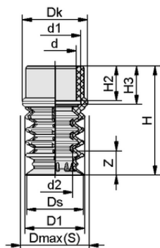
Конструктивные данные SPB4 20 SI-55 SC080
