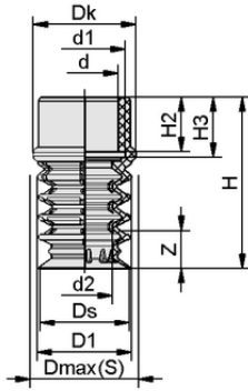
Tasarım verileri SPB4 20 SI-55 SC080
