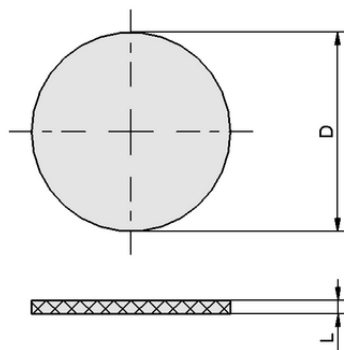
Конструктивные данные FD 16 120
