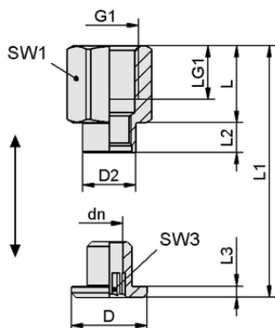
Konstruktionsdaten SC 040-AR G1/8-IG MOD
