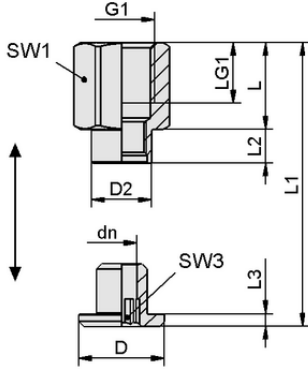
Tasarım verileri SC 040-AR G1/8-IG MOD
