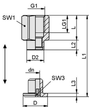
Конструктивные данные SC 040-AR G1/8-IG MOD
