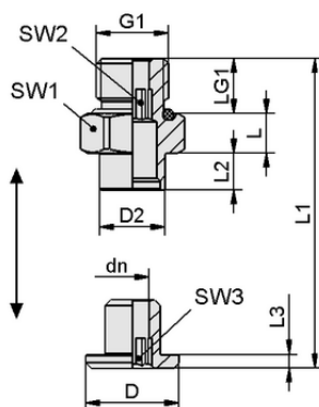
Конструктивные данные SC 040-AR G1/8-AG MOD
