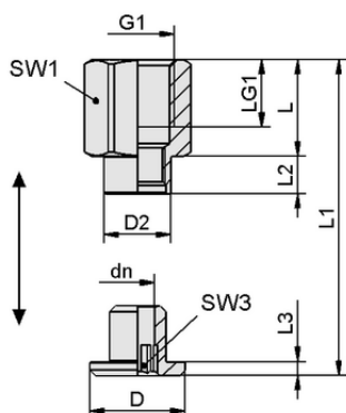
Конструктивные данные SC 050 G1/4-IG MOD
