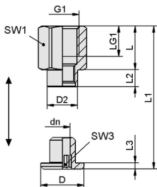
デザインデータ SC 050 G1/4-IG MOD
