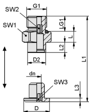
Конструктивные данные SC 050 G1/4-AG MOD
