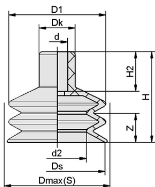
Конструктивные данные FG 50 PVC-50 N033
