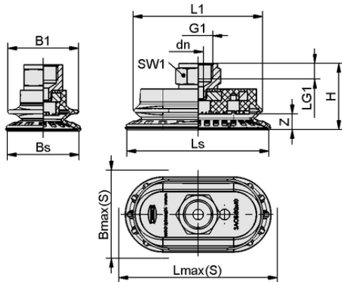
Datos de diseño SAOB 80x40 HT2-65 G1/4-IG
