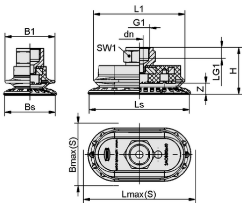
Données de construction SAOB 60x30 HT2-65 G3/8-IG
