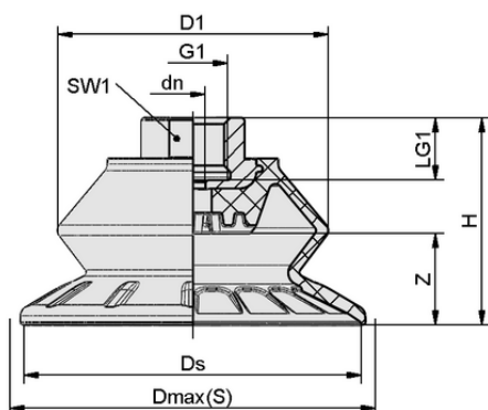
Dati di costruzione SAB 30 HT2-65 G1/4-IG
