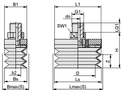
デザインデータ FSGB-R 52x25 SI-50 G1/4-AG
