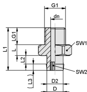
Конструктивные данные SA-NIP N058 G1/8-AG DN500
