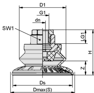
Datos de diseño SAB 80 NBR-60 NPT3/8-IG
