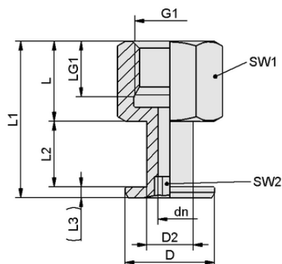
Dati di costruzione SA-NIP N019 G1/4-IG DN820
