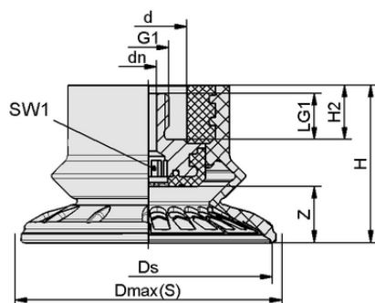
デザインデータ SABT-C 80 NBR-60 M10-AG
