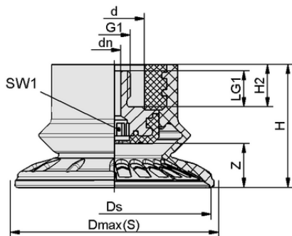
Données de construction SABT-C 60 NBR-60 M10-AG
