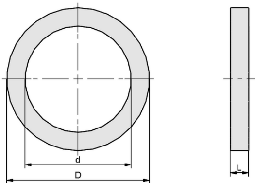
Design data DR 28/21x3 C03 EPDM-15 KE
