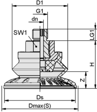
Tasarım verileri SAB 22 NBR-60 M14x1.5-AG
