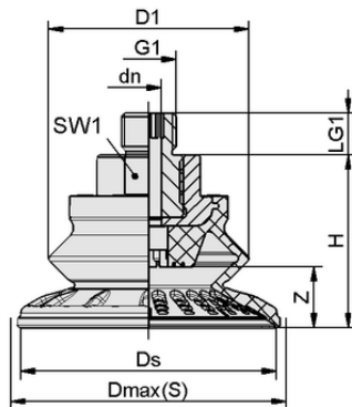
Données de construction SAB 22 NBR-60 M10-AG
