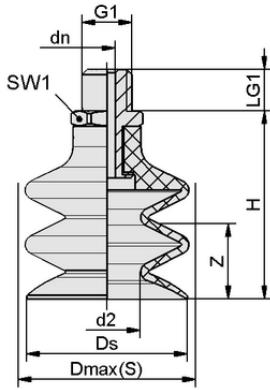
Tasarım verileri FSG 12 HT1-60 M5-AG
