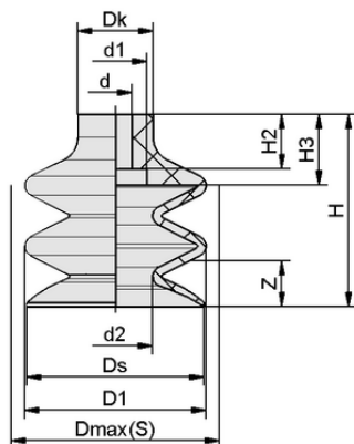
Données de construction FG 32 HT1-60 N018
