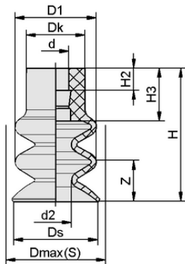
Datos de diseño FG 20 HT1-60 N016
